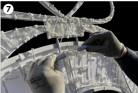
▲ リボンとリングの電源を連結します。
