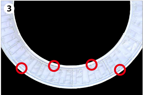
▲ 土台と同様にリング本体にも連結用の穴が4点ある事をご確認ください。
